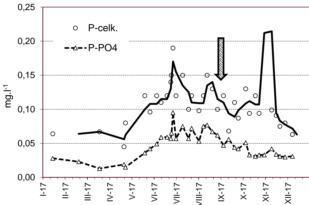
Mže Stříbro pod: koncentrace fosforu 2017
