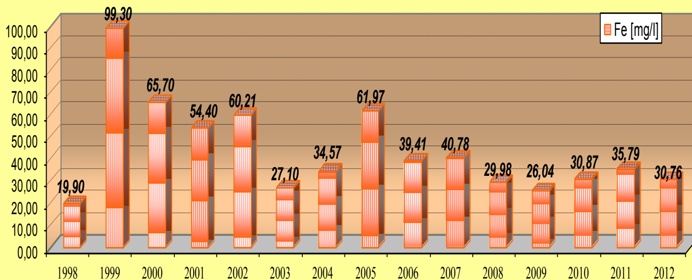
Vývoj průměrných koncentrací Fe v letech 2002 - 2012
