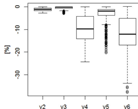
I během opatření NO 2 maximální 1h průměr
