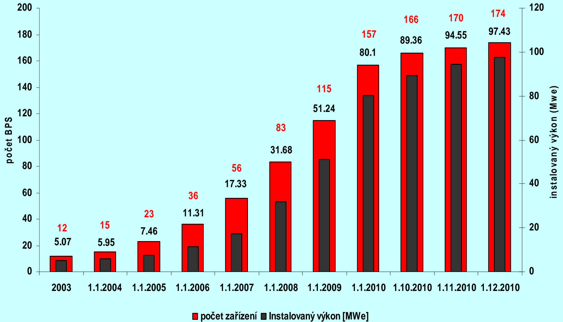
Počet a instalovaný výkon BPS v letech 2003 - 2010
