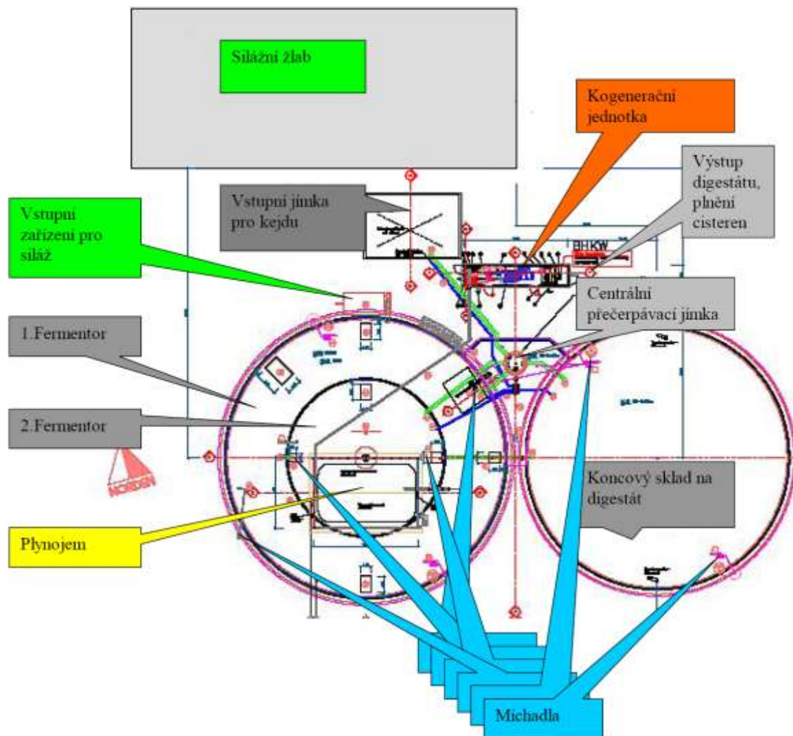
Schéma BPS AGRI FAIR s.r.o.
